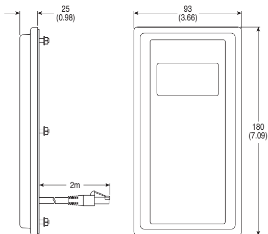
Рис. Б.13 Удаленный сокращенный модуль НИМ (крепление на панели). Размеры указаны в миллиметрах (в скобках даны значения в дюймах). Номер по каталогу: 22-НИМ-С2S
