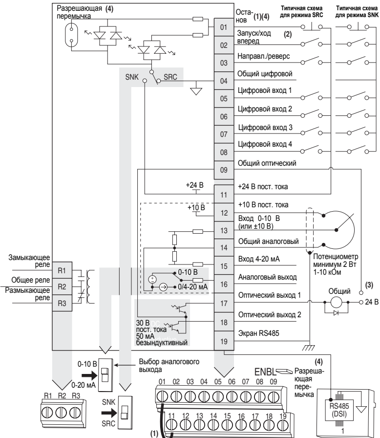
Рис. 1.5 Структурная схема цепей управления
